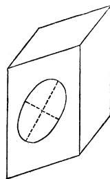
FIG. 7.—Augite (var. diopside).
